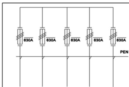
Układ sieci TN-C
