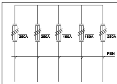
Układ sieci TN-C
