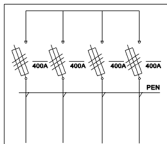
Układ sieci TN-C
