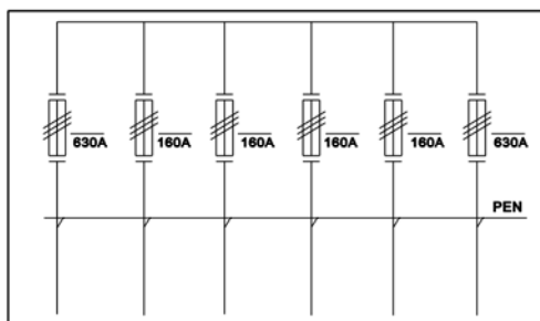
Układ sieci TN-C
